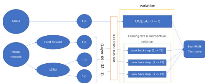
รูปที่ 4 ขั้นตอนในการทดสอบและคัดเลือกอัลกอริทึมในการศึกษา
