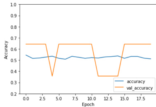
ภาพที่ 22 Accuracy result trend after 60 rounds training with learning rate 0.1
