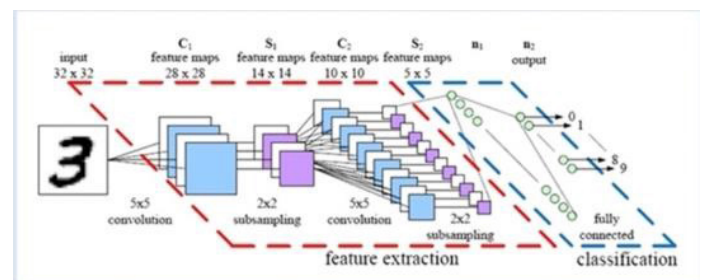
ภาพที่ 14 ภาพตัวอย่างการทำ Architecture Model CNN
